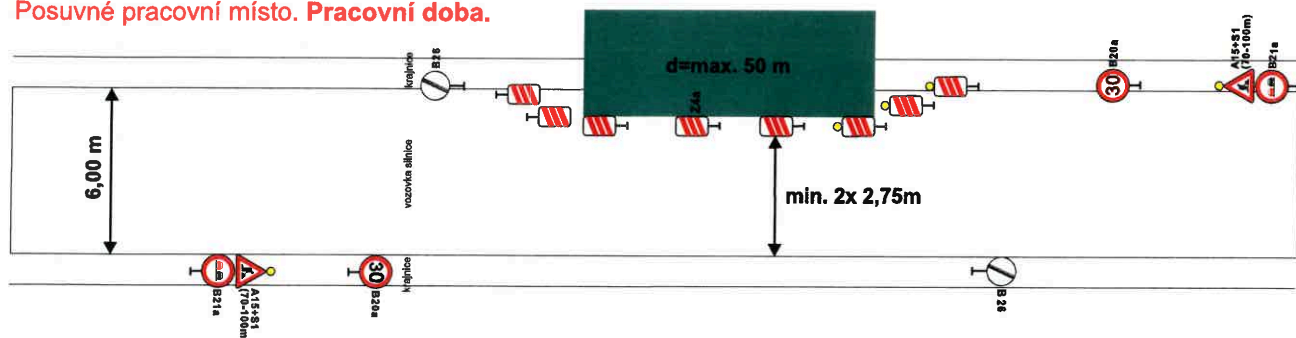
DETAIL 2- schéma pracovního místa na silnici III/02019. Posuvné pracovní místo. Pracovní doba.
