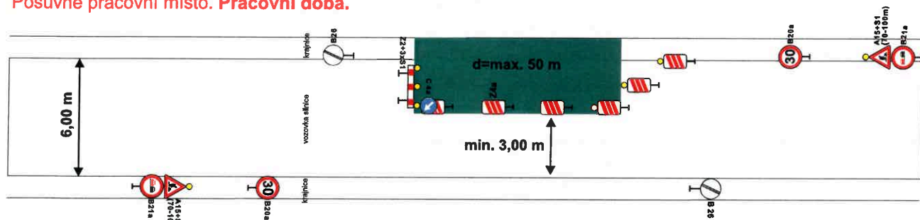
DETAIL 2- schéma pracovního místa na silnici III/02019. Posuvné pracovní místo. Pracovní doba.
