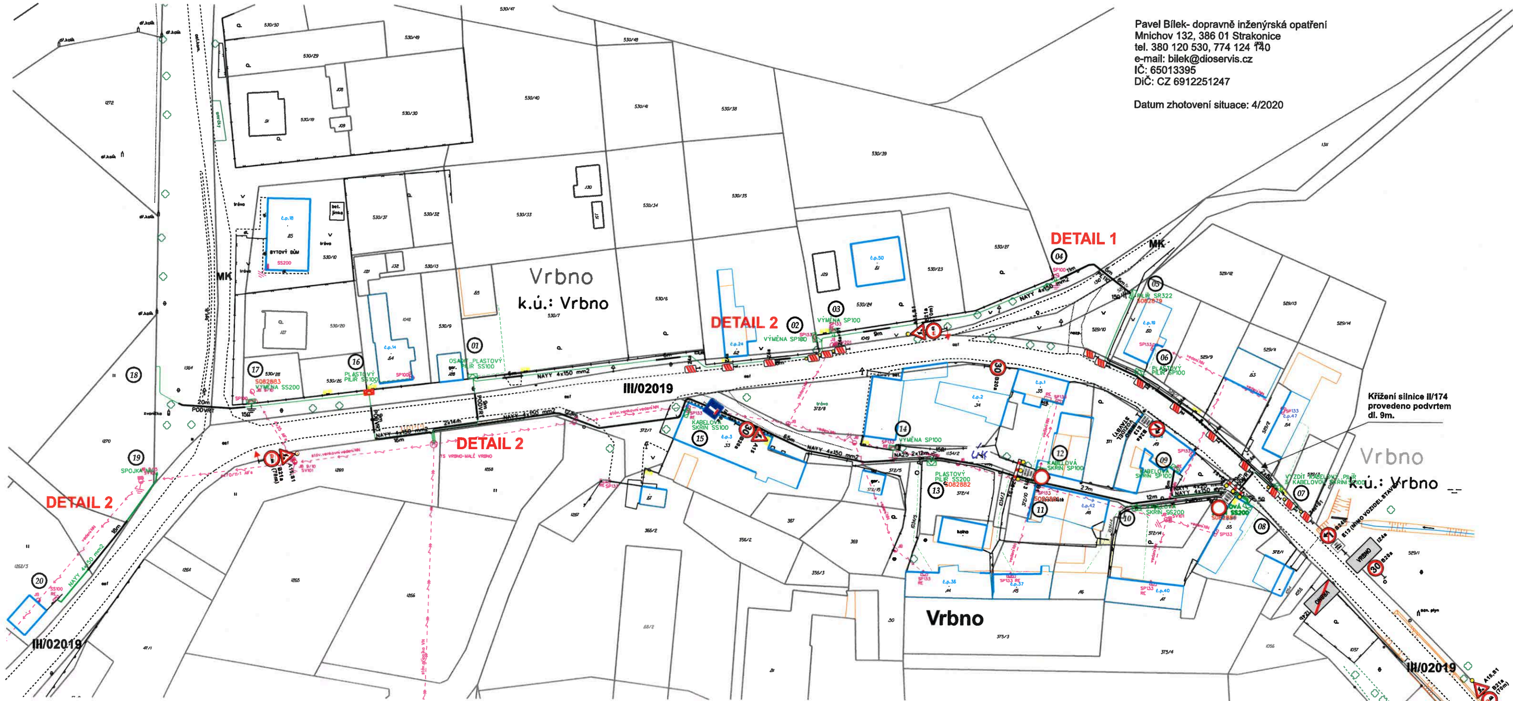
DETAIL 1- schéma pracovního místa na silnici III/02019 a u místa komunikací. Posuvné pracovní místo. Pracovní doba.
